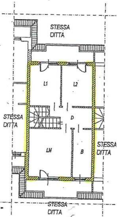
PIANTA PIANO PRIMO h=2.70 m
