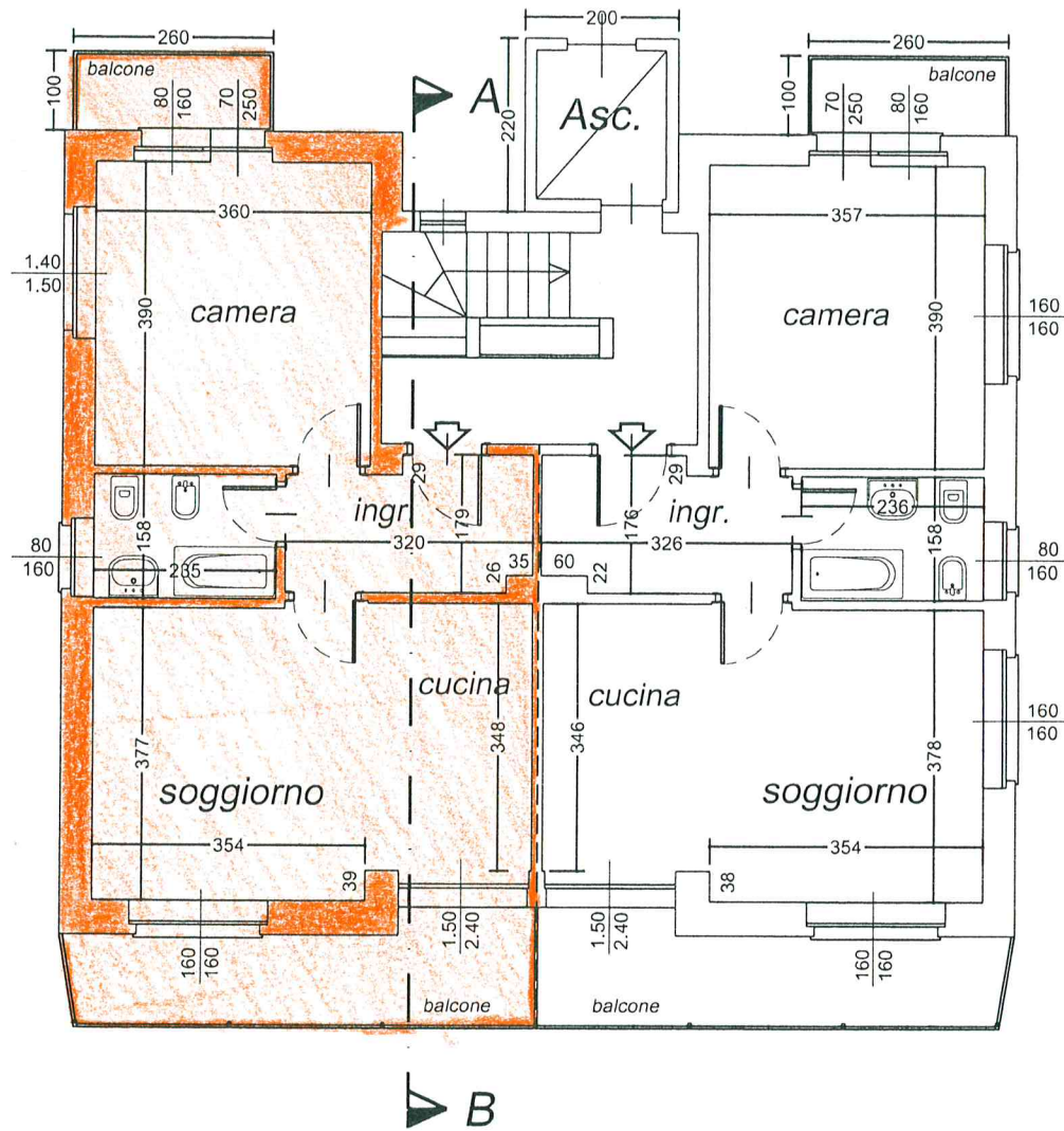
PIANTA PIANO TERZO
